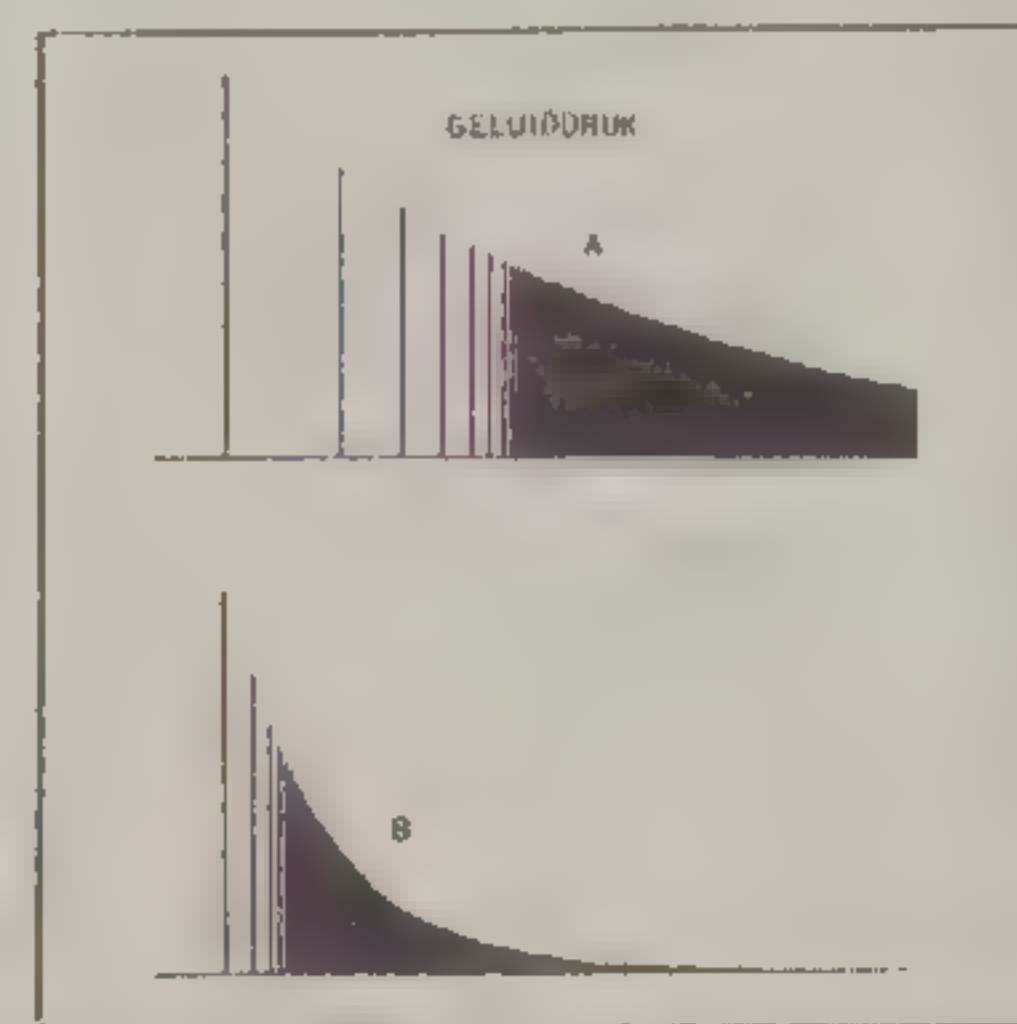
fig. 6 Pulsresponsies van concertzaal (A) en huiskamer (B)
